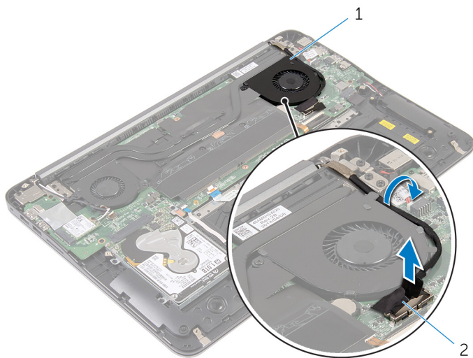
1 处理器风扇
